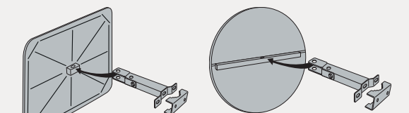
sur poteau / sur mur fixation en acier inoxydable
